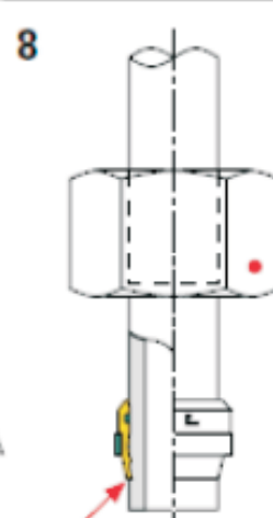
Проверка врезного кольца
